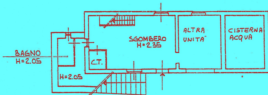
PIANTA PIANO SEMINTERRATO
